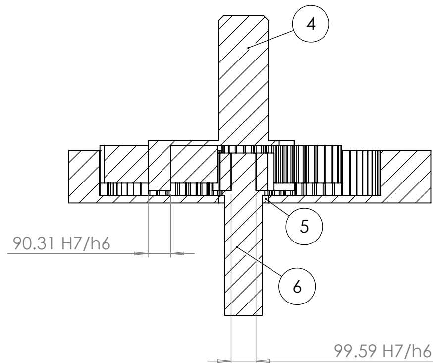
SECTION A-A SCALE 1 : 15
