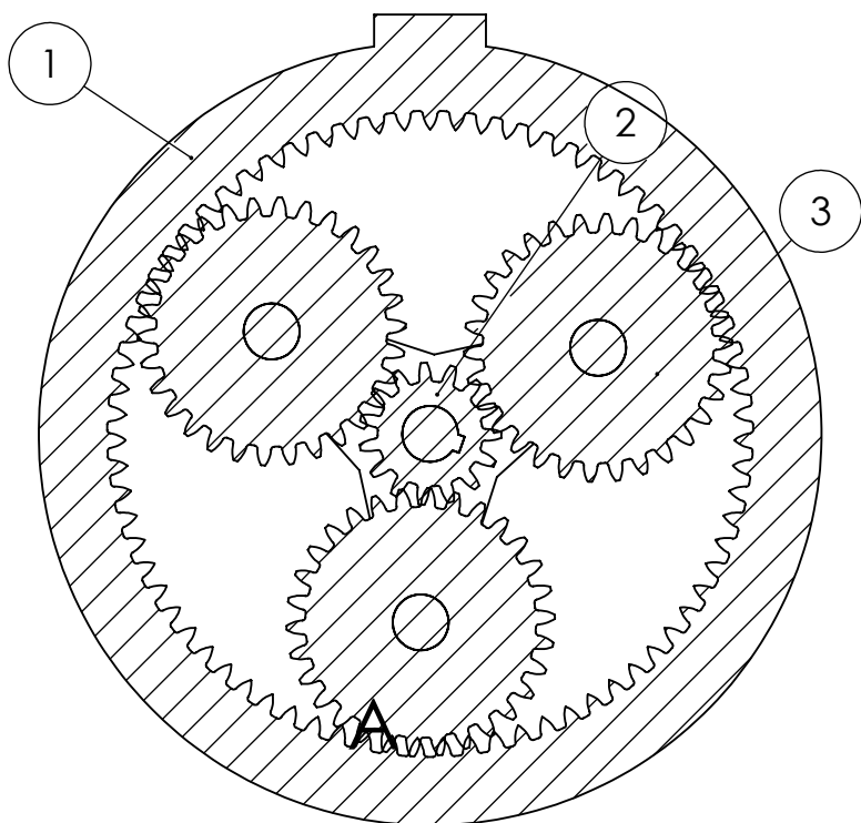
SECTION B-B SCALE 1 : 15
